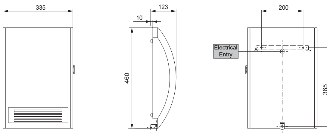
CK / CKZ Dimensions
